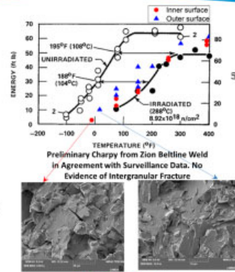
Fig. 1 Zion RPV testing
